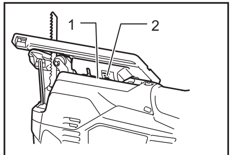
► 1. Borde 2. Graduación
