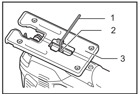
► 1. Llave hexagonal 2. Tornillo 3. Base
