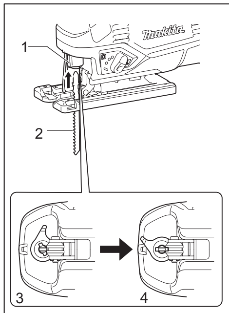
► 1. Porte-lame 2. Fer 3. Position d'immobilisation 4. Position ouverte
