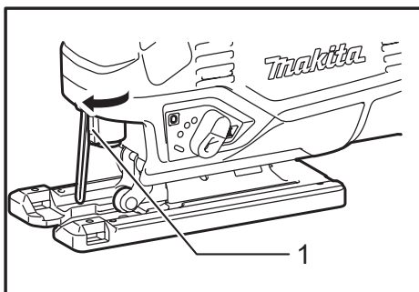
► 1. Levier de serrage de la lame
